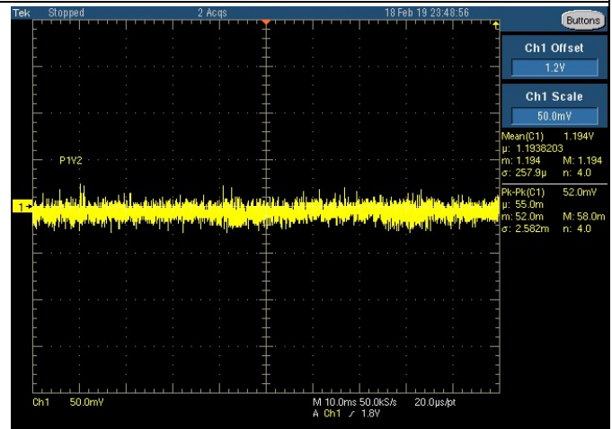
Fig. 8: P1V8
